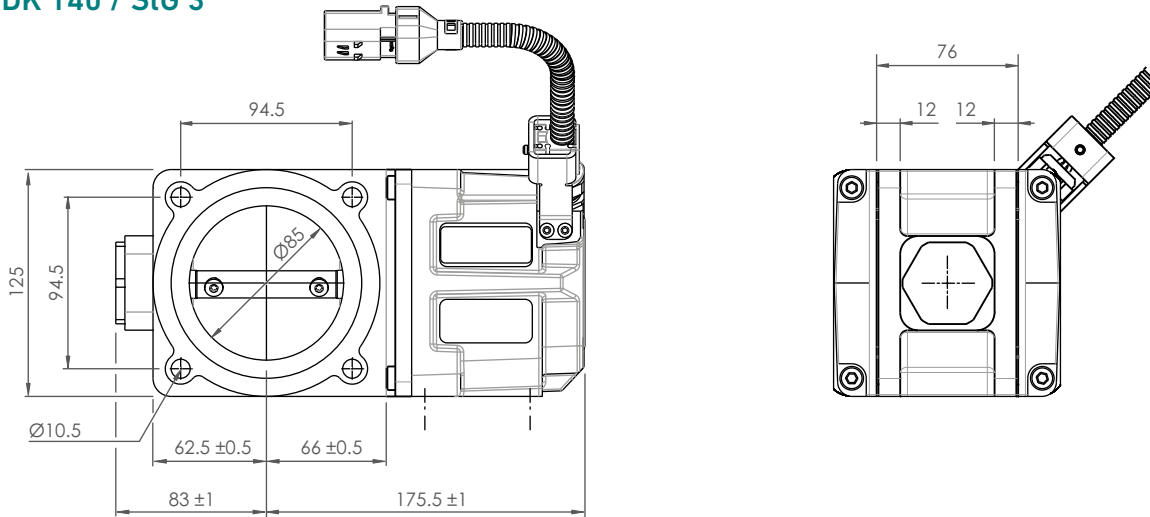
DK 140 - Dichtung, Artikel-No.: 463-24-000-00
