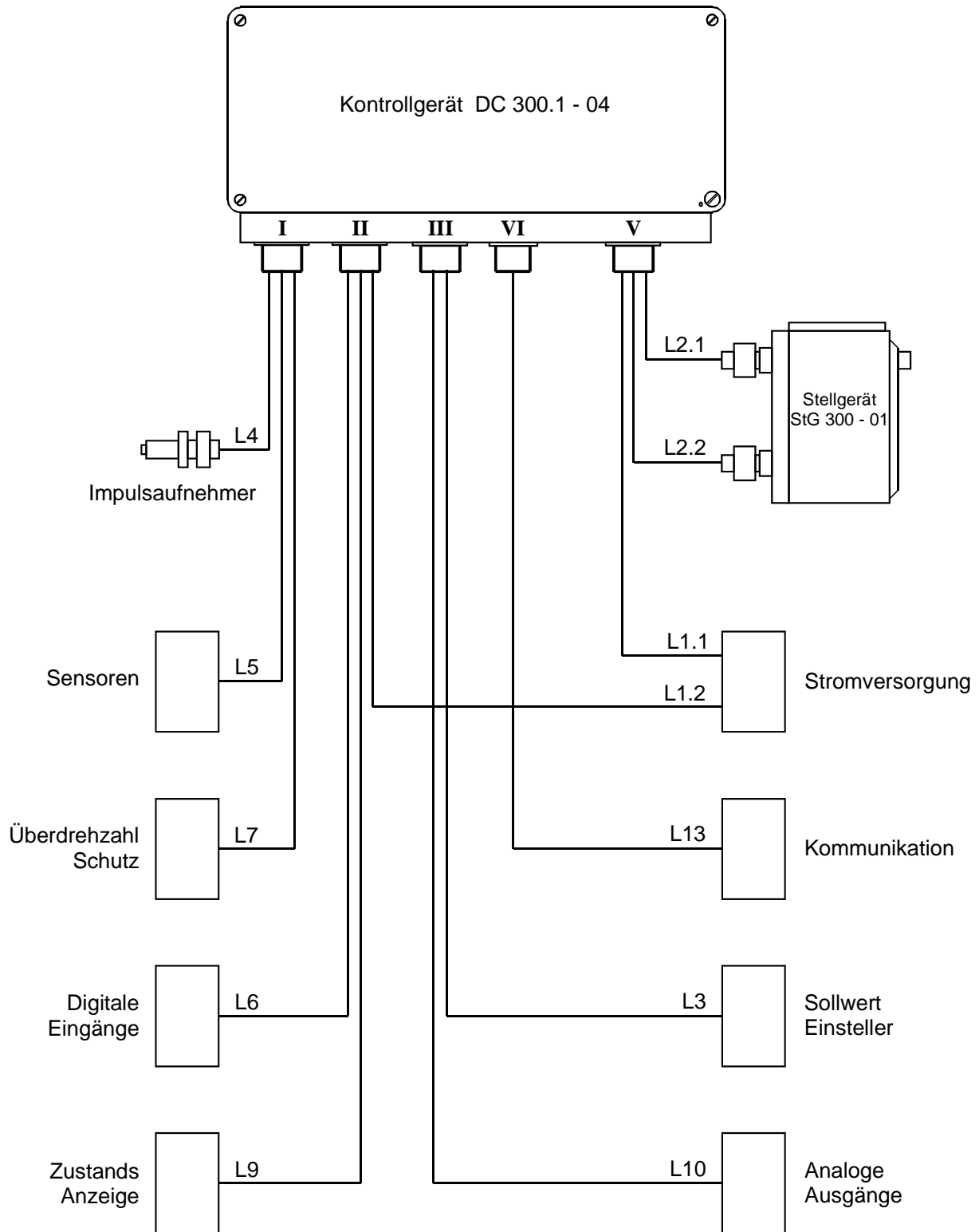
Abbildung 20: Kabelbaum mit Kabelbezeichnungen
