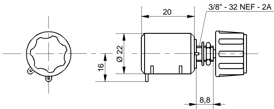
Abbildung 9: Potentiometer SW 02 - 10
