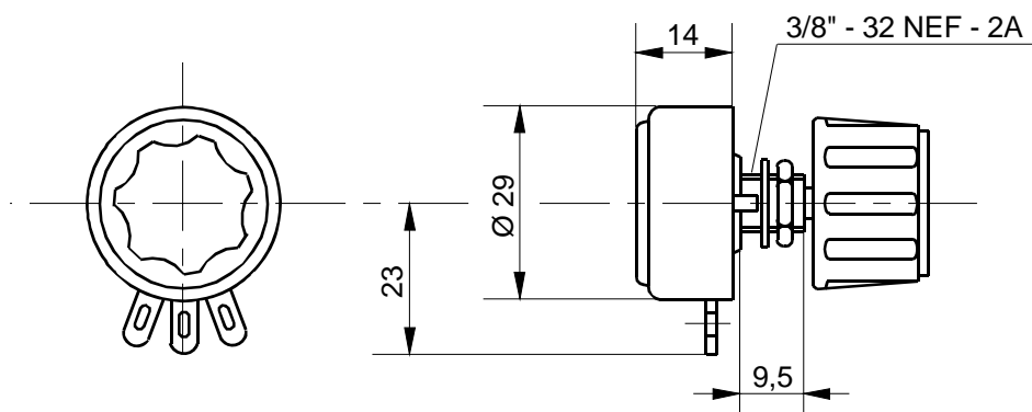
Abbildung 8: Potentiometer SW 01 - 1
