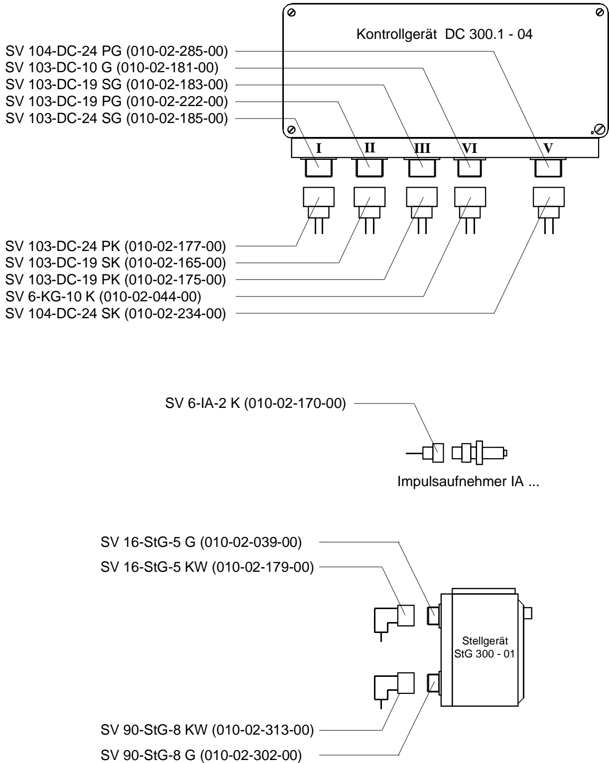
Abbildung 21: Gehäuse mit Steckerbezeichnungen
