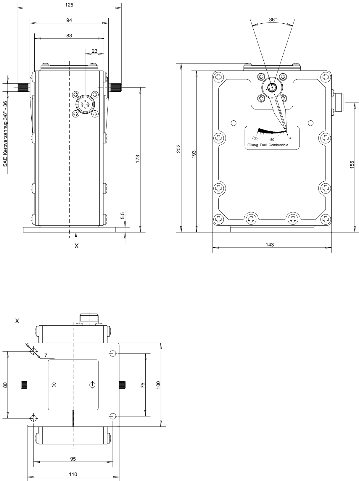
Abbildung 8: Maßzeichnung StG 10-01
