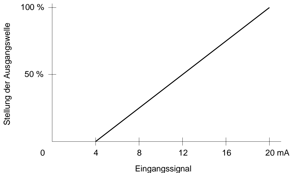
Abbildung 1: Zusammenhang zwischen Eingangssignal und Position
