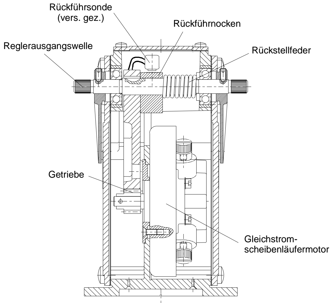
Abbildung 5: Prinzip Stellgeräte (Beispiel StG 6-01)
