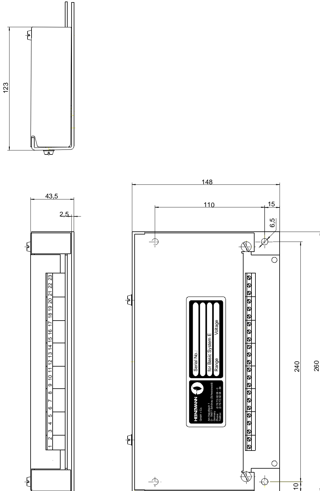
Abbildung 4: Maßzeichnung PKG .. - 04 - 00
