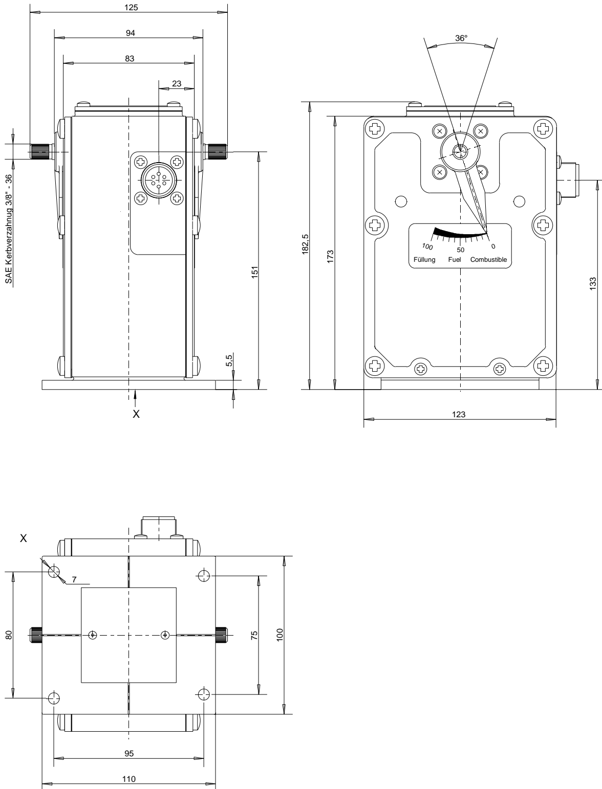
Abbildung 7: Maßzeichnung StG 6-01 und StG 6-02 V
