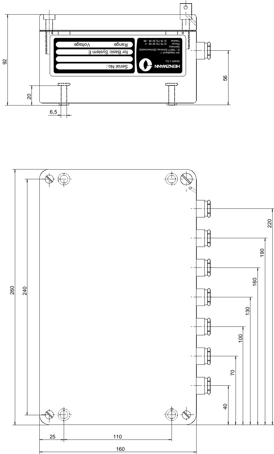
Abbildung 3: Maßzeichnung PKG .. - 04 - 55
