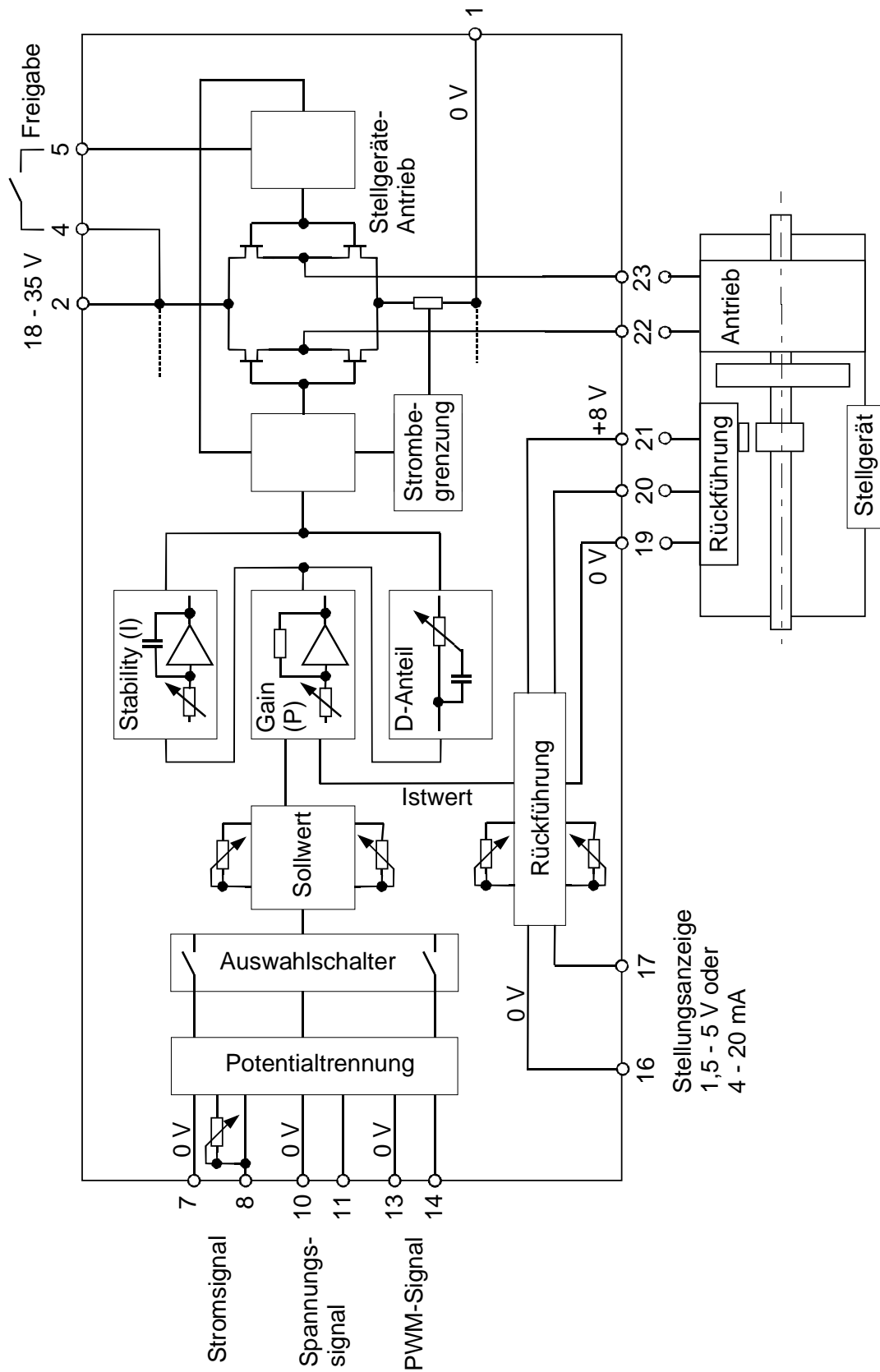
Abbildung 2: Blockschaltbild
