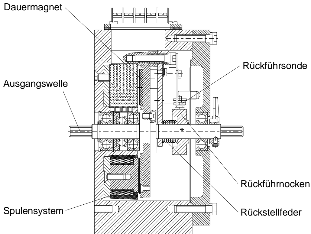
Abbildung 6: Prinzip StG 2010-01 bis 2080-01
