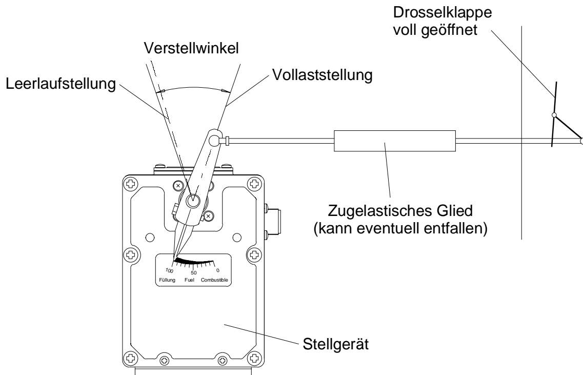
Abbildung 14: Gestänge für Gasmotoren
