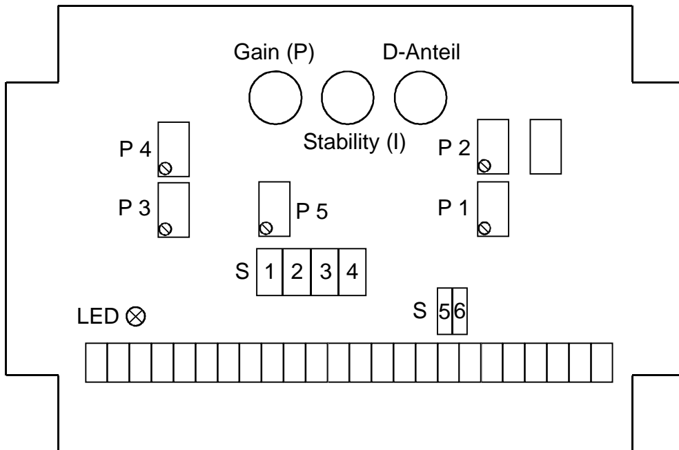
Abbildung 17: Einstellungsschalter und Potentiometer PKG .. - 04
