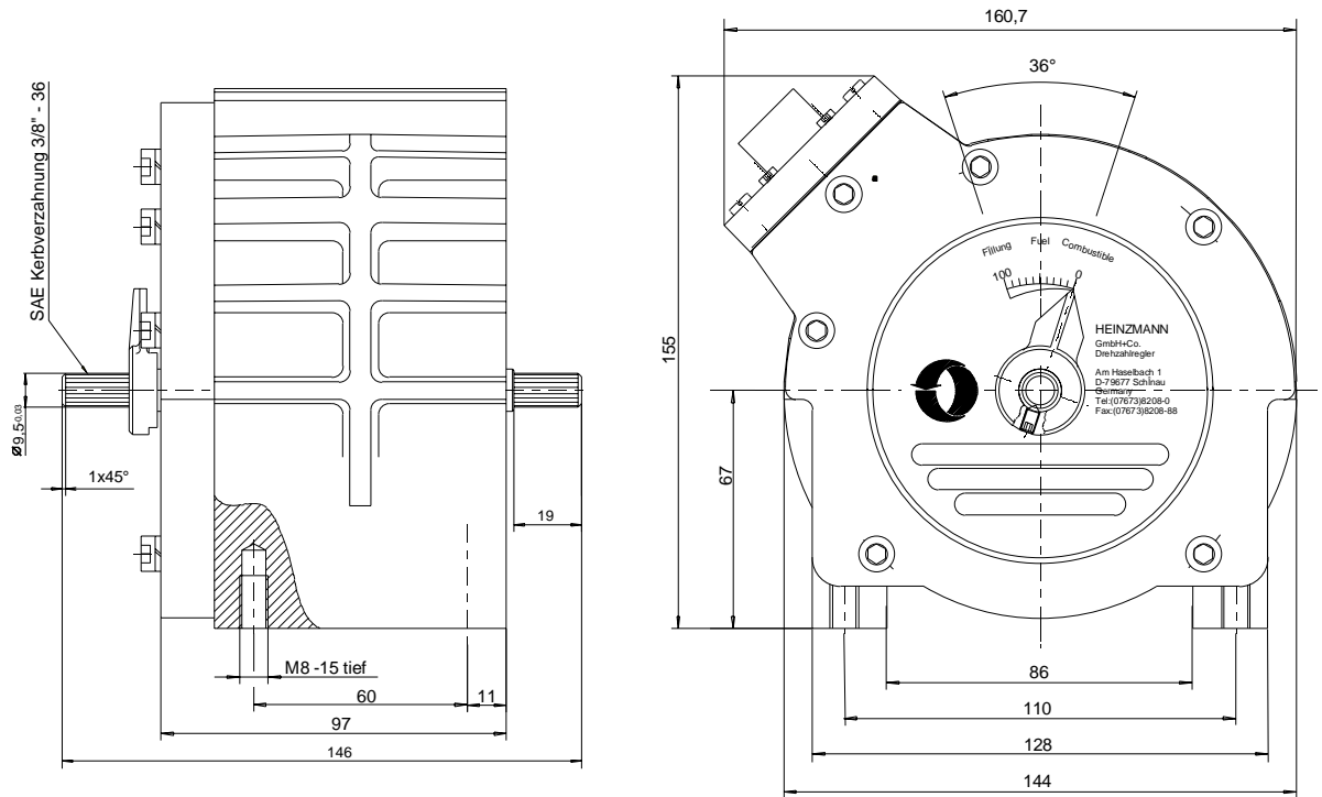
Abbildung 11: Maßzeichnung StG 2040-01
