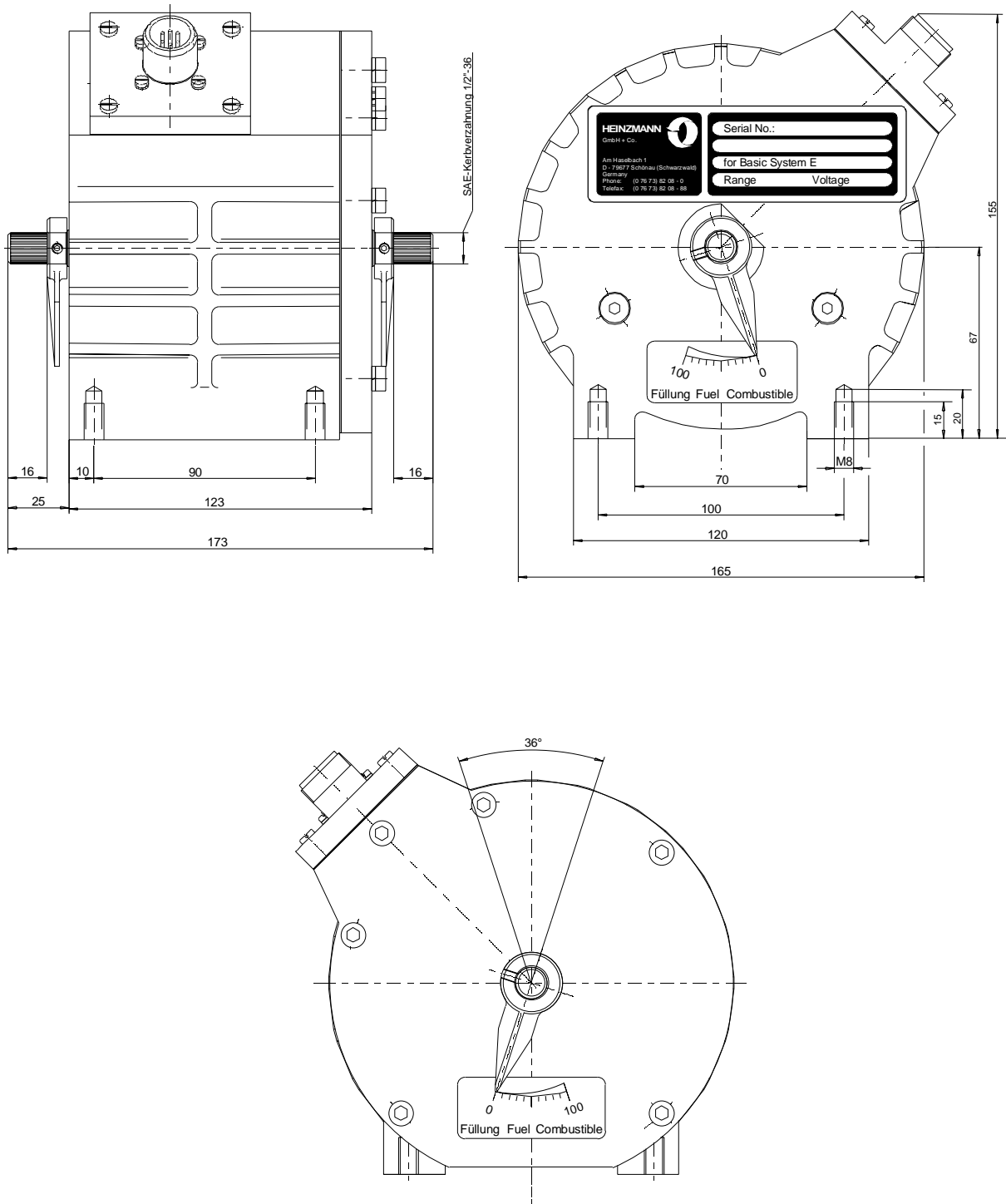
Abbildung 12: Maßzeichnung StG 2080-01
